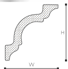
A1 NOMASTYL® H 80 x W 80 mm Face Dim. 113 mm
