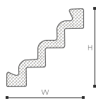
ST3 NOMASTYL® H 75 x W 75 mm Face Dim. 106 mm
